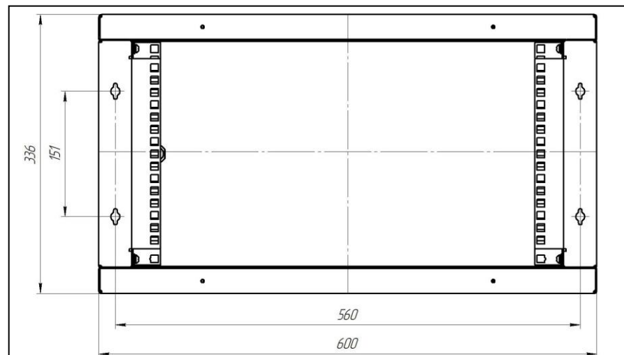
Рисунок 2 – Установочные размеры серверного шкафа
