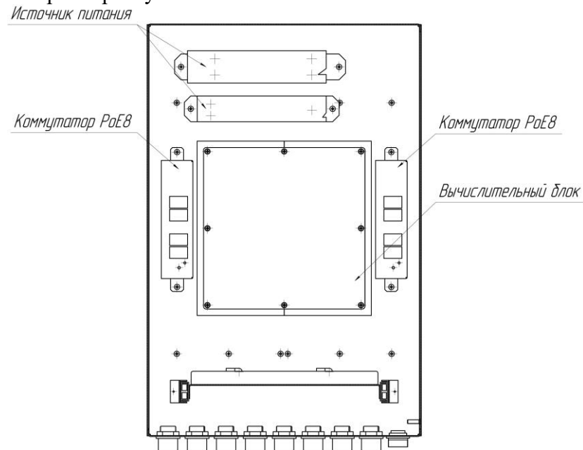
Рисунок 1 – Контроллер STS-422 без двери и панели с монитором
