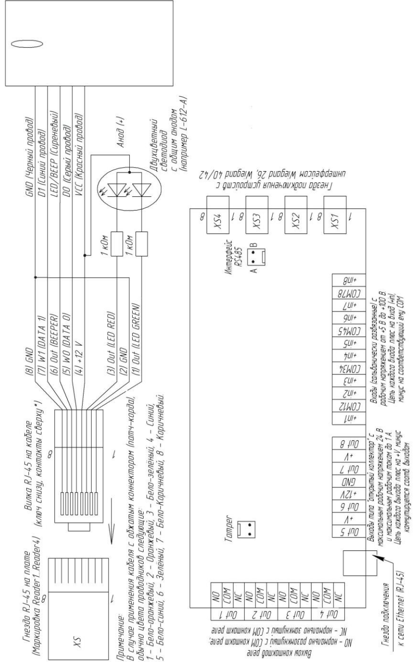
Рисунок 2 – Подключение контроллера STS-408
