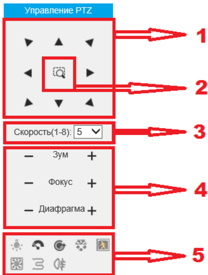
Рисунок 9 - Конфигурации PTZ
