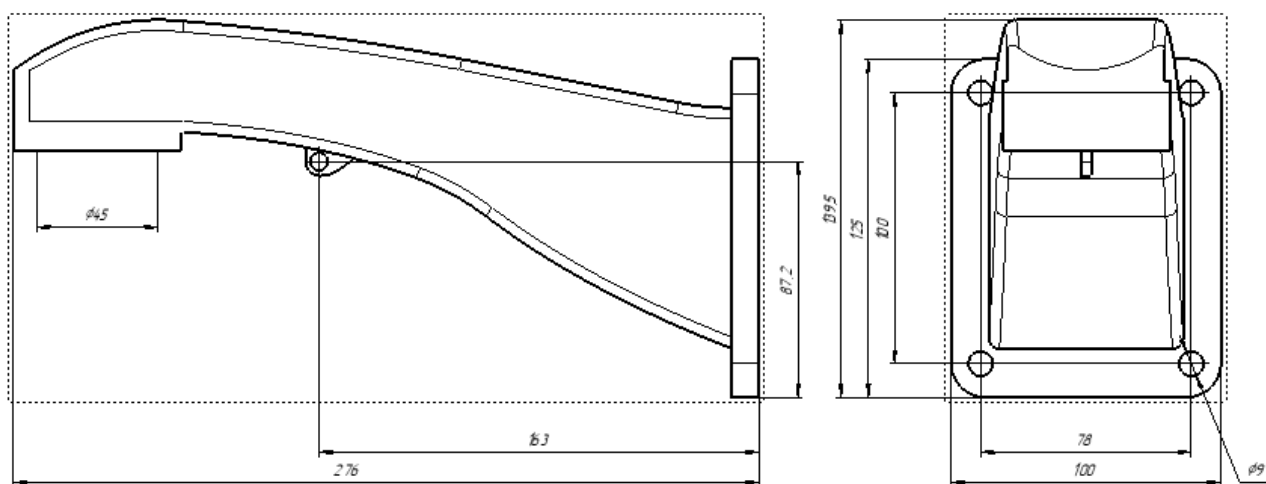
Рисунок 3 – Габаритные размеры кронштейна IP-видеокамеры TBS-UP
