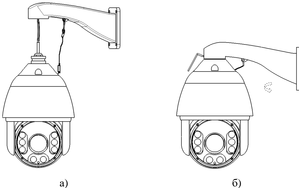
Рисунок 6 - Установка видеокамеры на кронштейне
