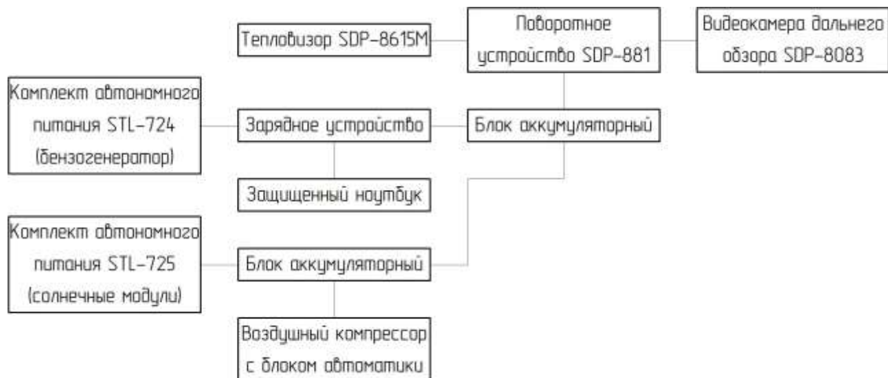
Рисунок 1.2 – Схема построения АМКВТН «Муром ВК» при использовании мачты STS-10903
