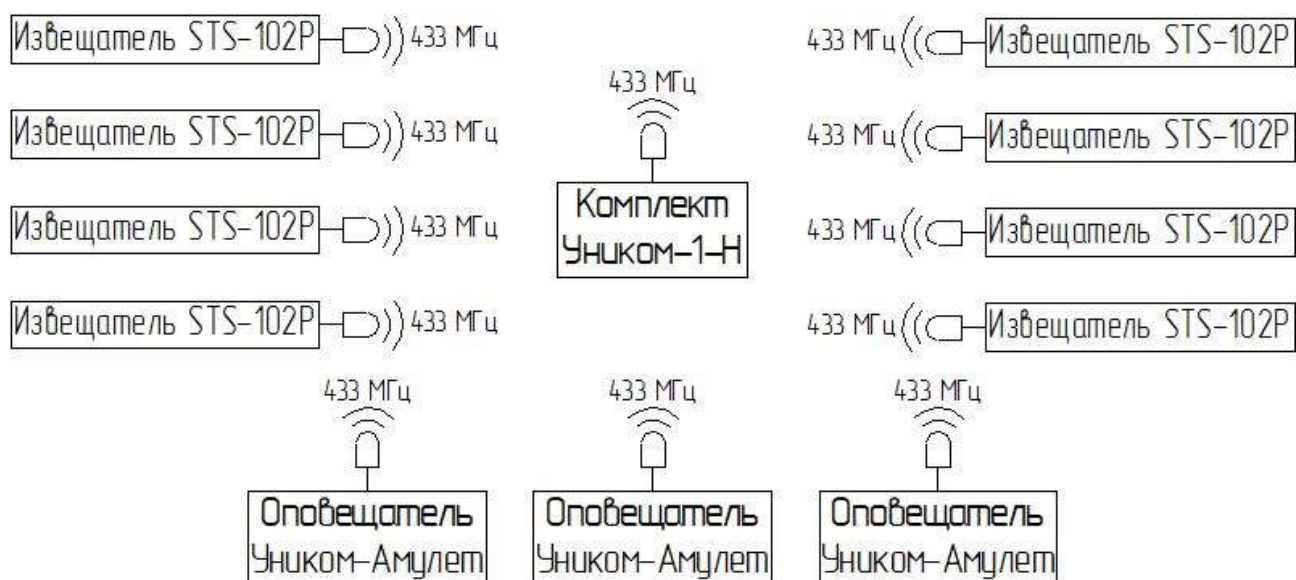
Рисунок 1.4 – Схема построения МКОУМ «Мангуст ВК» при самостоятельном использовании (отдельно от АМКВТН «Муром ВК»)
