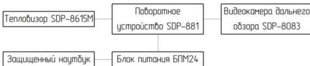
Рисунок 1.3 – Схема построения АМКВТН «Муром ВК» при использовании мачты STS-10901
